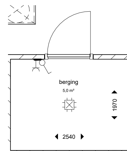
berging 1 : 50
