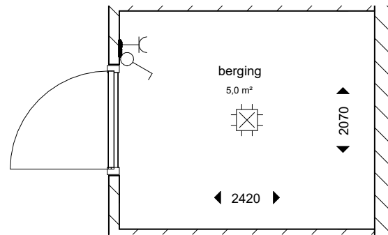
berging 1 : 50
