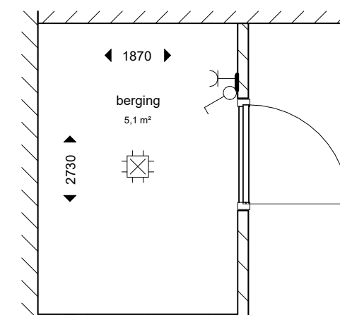
berging 1 : 50
